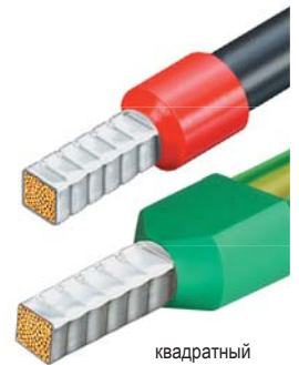
квадратный обжим
