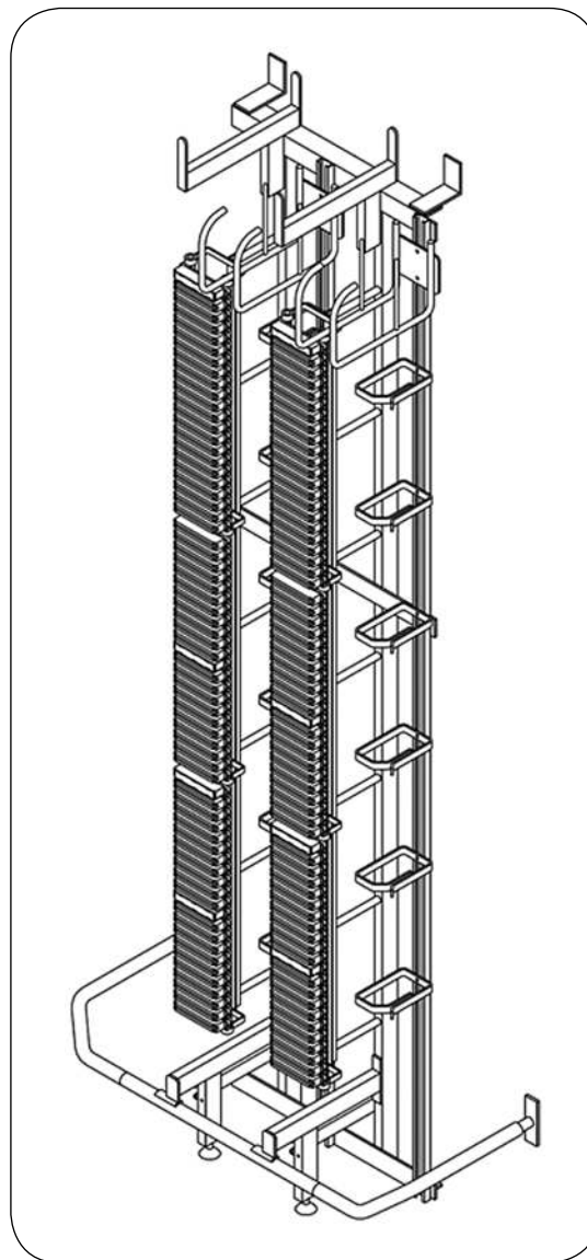
Оснащенный главный кросс типа 91M с рамами PROFIL (глубина 46 мм)
