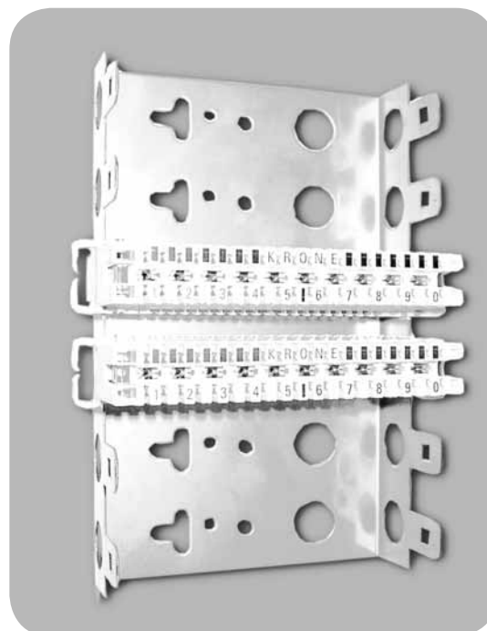
Монтажный хомут R (растр) = 27,5 мм для 6 плиток (плитки не входят в состав поставки)
