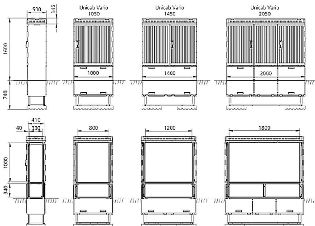
Габаритные размеры корпусов распределительного шкафа типа Unicab-Vario
