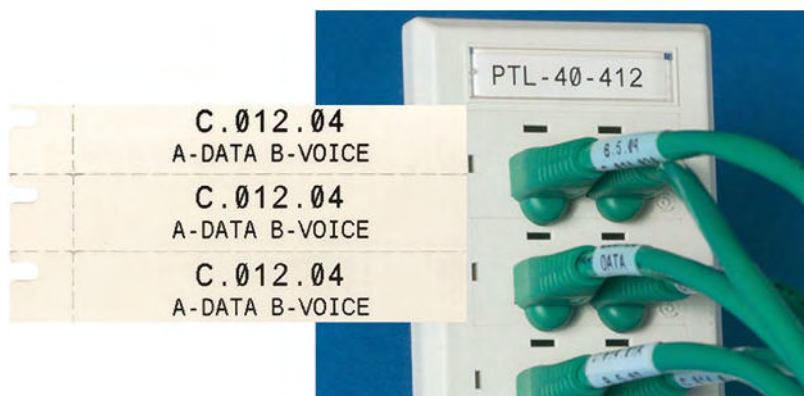
Рис. 6-9. Примеры этикеток «Маркировочная полоса»
