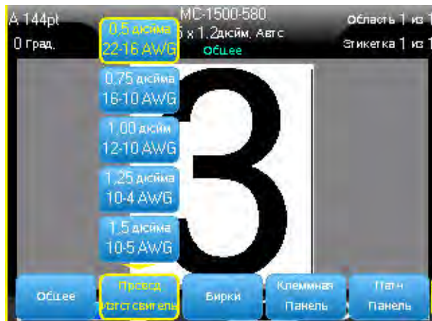
Рис. 6-2. Повторение данных на этикетке маркера проводов и маркера кабелей
