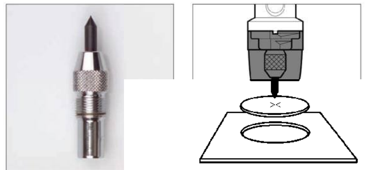
Держатель резака
