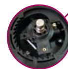
16-зубцовый механизм фиксации с возвратной пружиной
