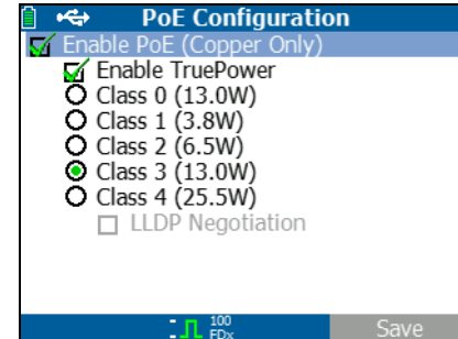
Рис.20. Конфигурация PoE на тестере LR-AT 2000
