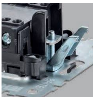
Анкерное крепление с фиксацией.
