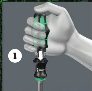
1 Механизм с разжимающей пружиной
