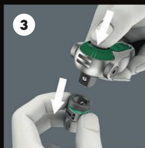
3 Шариковый фиксатор
