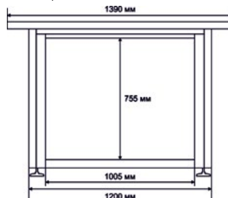
Верстак под 2 модуля вид спереди
