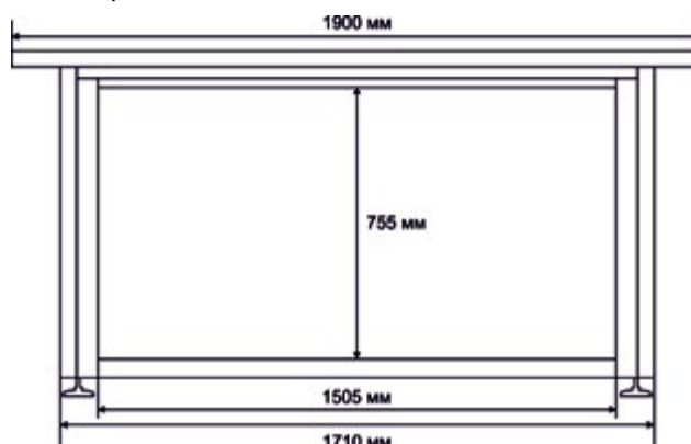
Верстак под 3 модуля вид спереди
