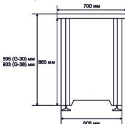
Верстак под модуль вид сбоку
