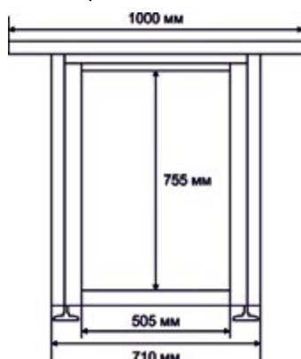
Верстак под 1 модуль вид спереди
