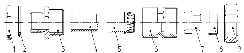
1 – Гайка крепежная 4 – Уплотнитель кабеля 7 – Оконцеватель металлорукава 2 – Кольцо уплотнительное 5 – Зажим фиксирующий 8 – Уплотнитель металлорукава 3 – Корпус 6 – Корпус кабельного ввода 9 – Гайка накидная
