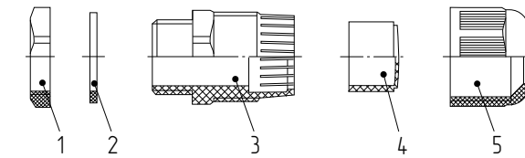
1 – Гайка крепежная 2 – Кольцо уплотнительное 3 – Корпус кабельного ввода 4 – Уплотнитель кабеля 5 – Гайка накладная
