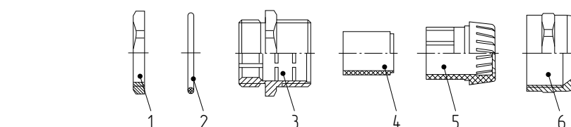
1 – Гайка крепежная 2 – Кольцо уплотнительное 3 – Корпус кабельного ввода 4 – Уплотнитель кабеля 5 – Зажим фиксирующий 6 – Гайка накидная
