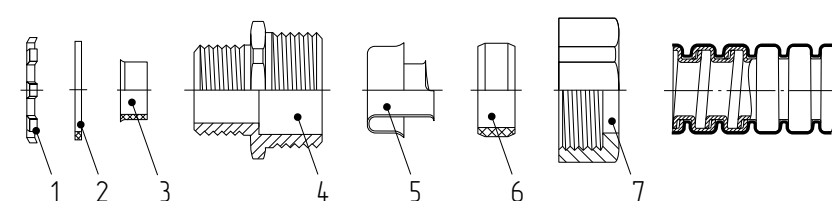
1 – Гайка заземляющая 2 – Кольцо уплотнительное 3 – Втулка защитная 4 – Корпус 5 – Оконцеватель металлокабеля 6 – Уплотнитель металлокабеля 7 – Гайка накидная
