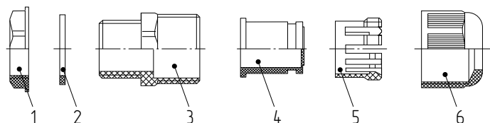
1 – Гайка крепежная 3 – Корпус кабельного ввода 5 – Зажим фиксирующий 2 – Кольцо уплотнительное 4 – Уплотнитель кабеля 6 – Гайка накладная
