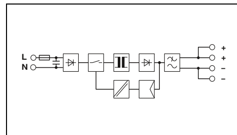
Источник питания, 1-фазный, 48 В DC, 100 Вт
