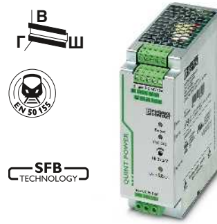
Преобразователь постоянного тока, с защитным покрытием, 96 – 110 В DC / 24 В DC, 10 А
