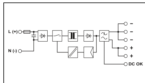
Источник питания, 1-фазный, 24 В DC, 4 А
