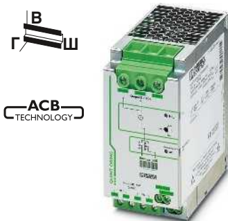
Активный модуль резервирования 24 В DC, 2x 40 А, 80 А
