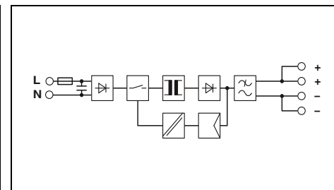
Источник питания, 1-фазный, 5 В DC, 40 Вт
