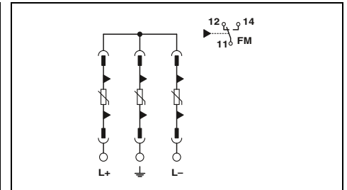
Штенерное устройство защиты от перенапряжения и тока молнии для ФГ-приложений до 1000 В пост. тока
