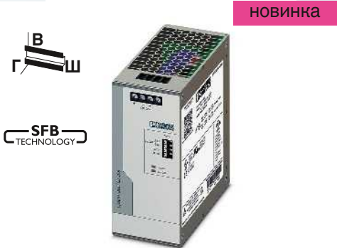
Необслуживаемый ёмкостный модуль 24 В DC / 20 А
