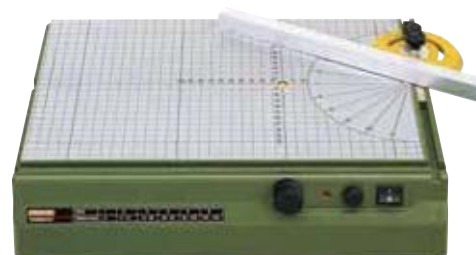
Поворотная направляющая со шкалой и фиксатором. (Немецкий патент 100 00 102.5)
