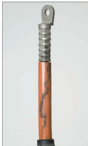
Образец, подвергшийся воздействию окружающей среды
